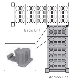
Add-on Unit
